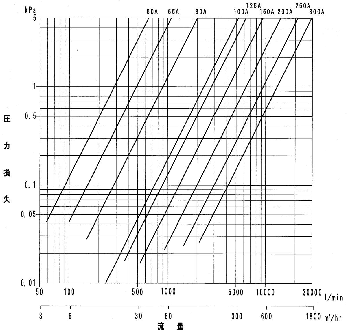
圧力損失-流量線図
