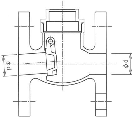
呼び径 25以下 本体形状
