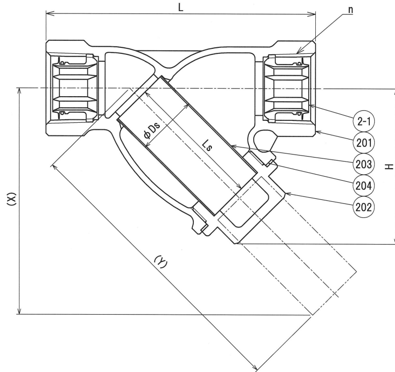
本体表示例(呼び径 3/4)
