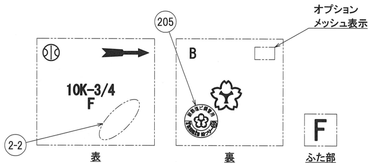
本体表示例(呼び径 3/4)
