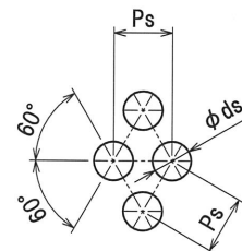
スクリーン詳細図
