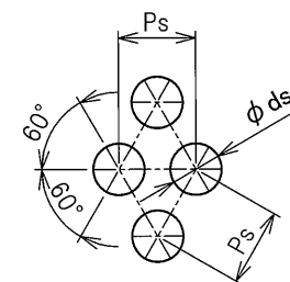
スクリーン詳細図
