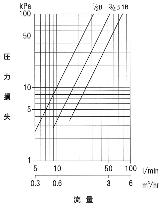
圧力損失—流量線図
