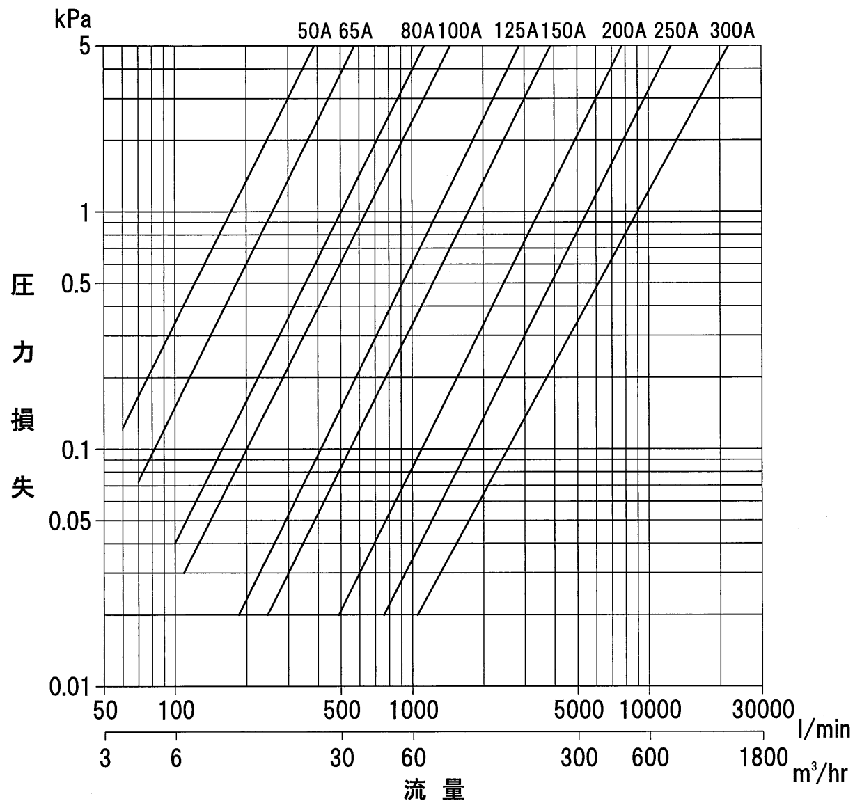
圧力損失—流量線図
