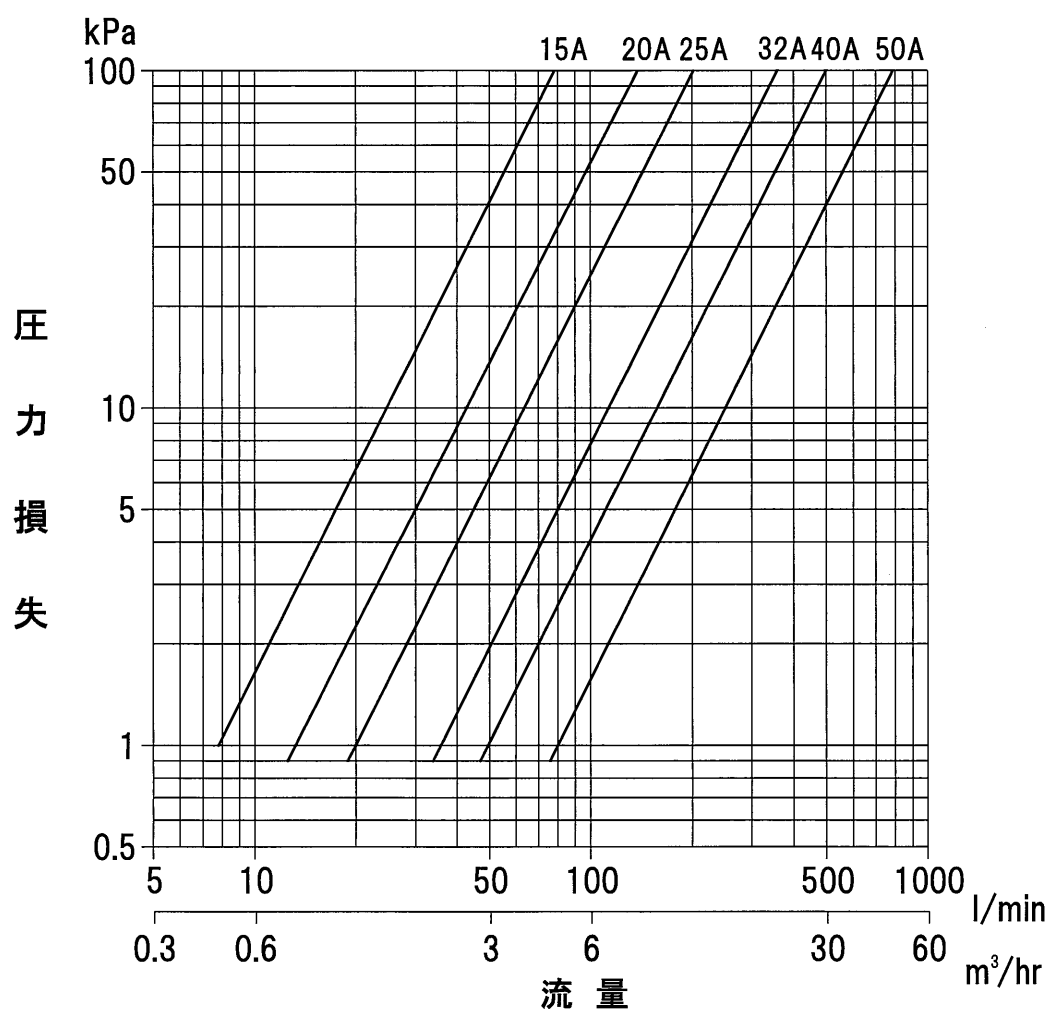
圧力損失—流量線図
