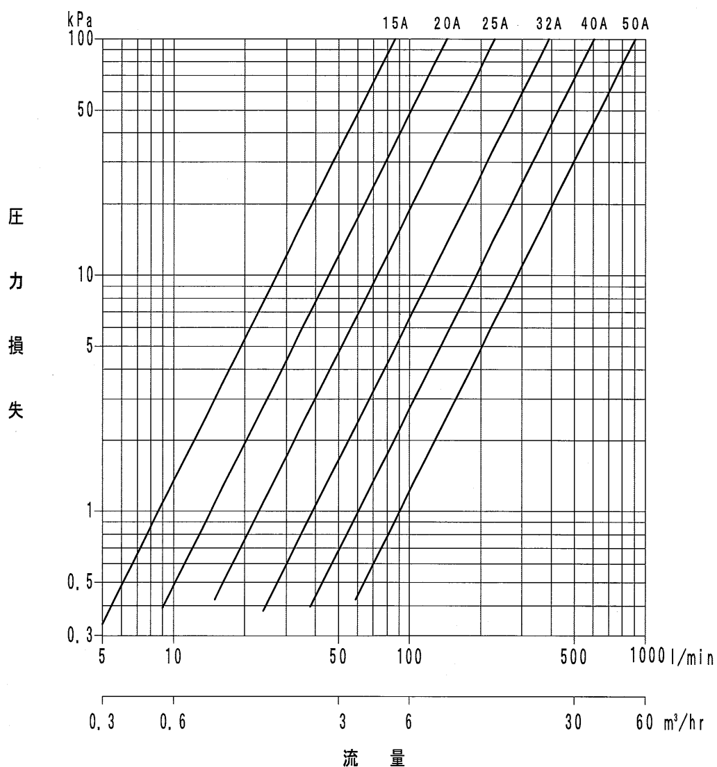
圧力損失-流量線図
