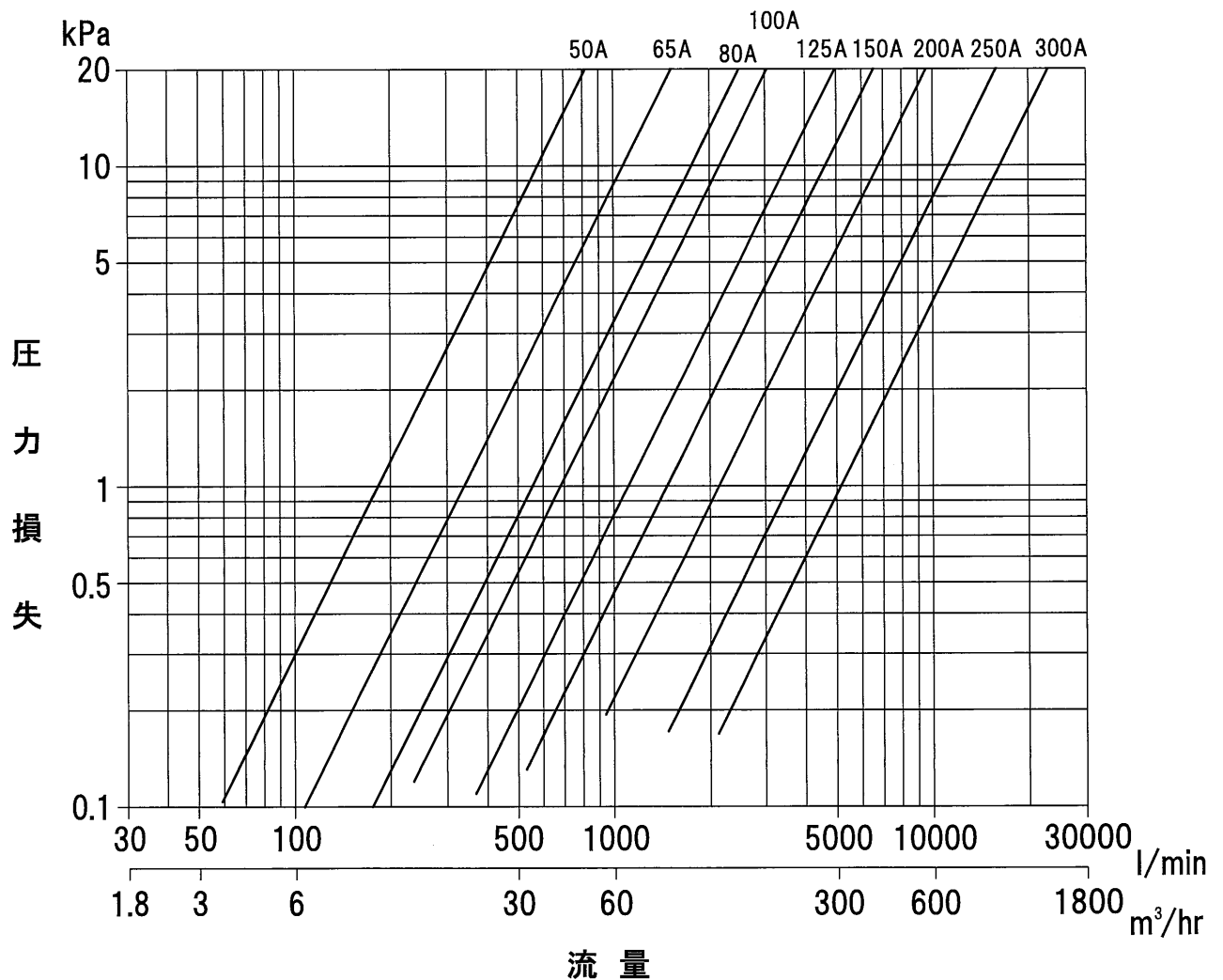
圧力損失—流量線図
