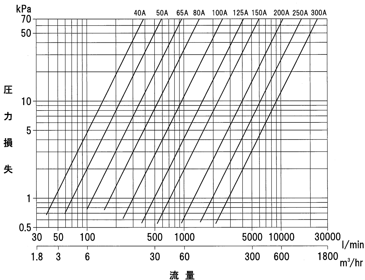
圧力損失－流量線図
