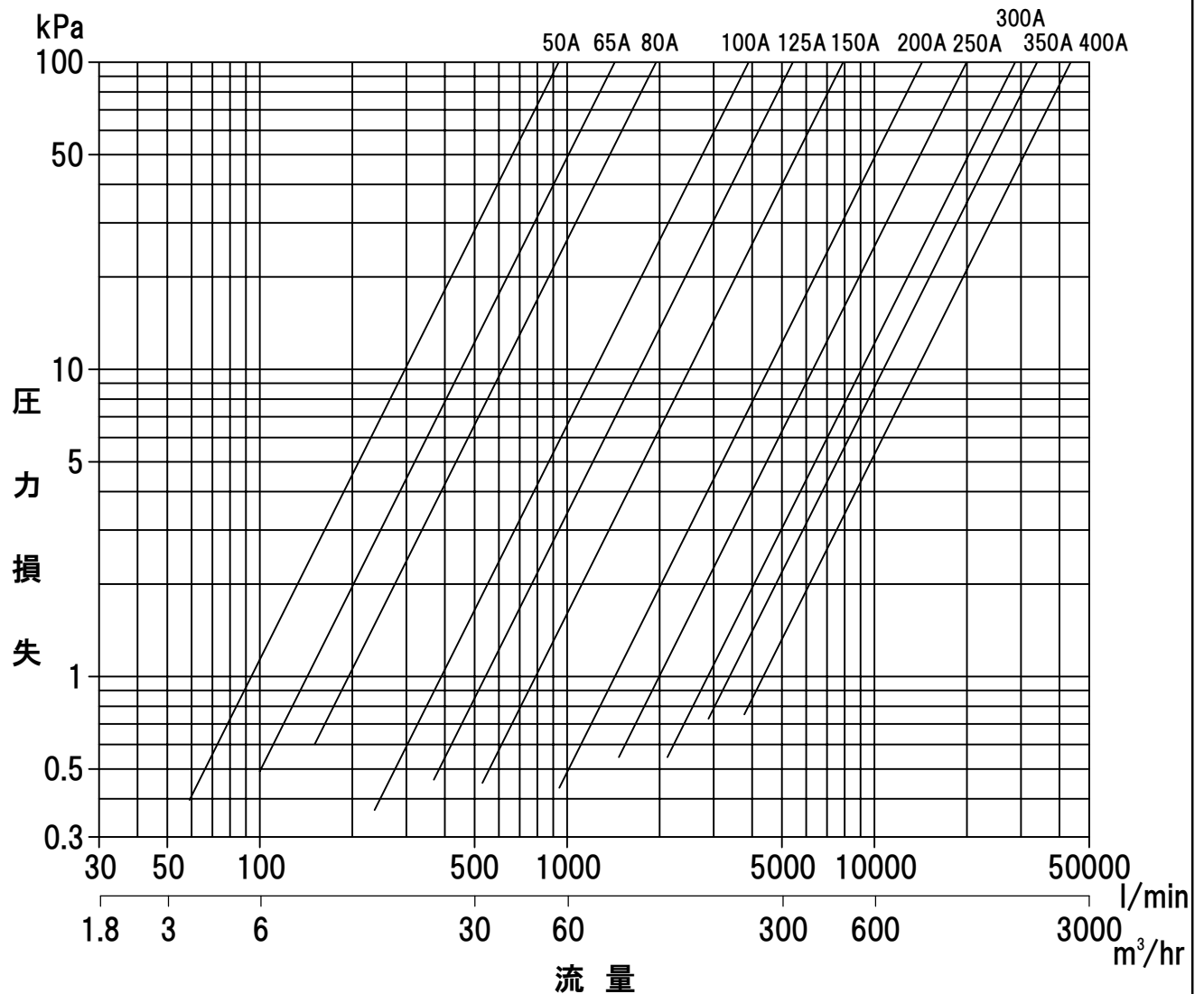
圧力損失—流量線図
