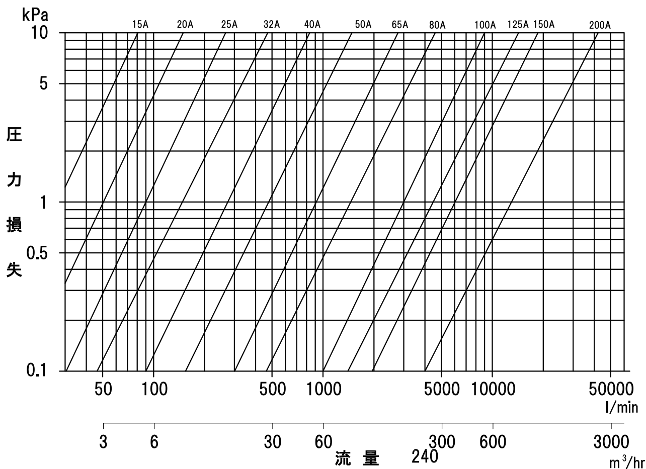
圧力損失—流量線図
