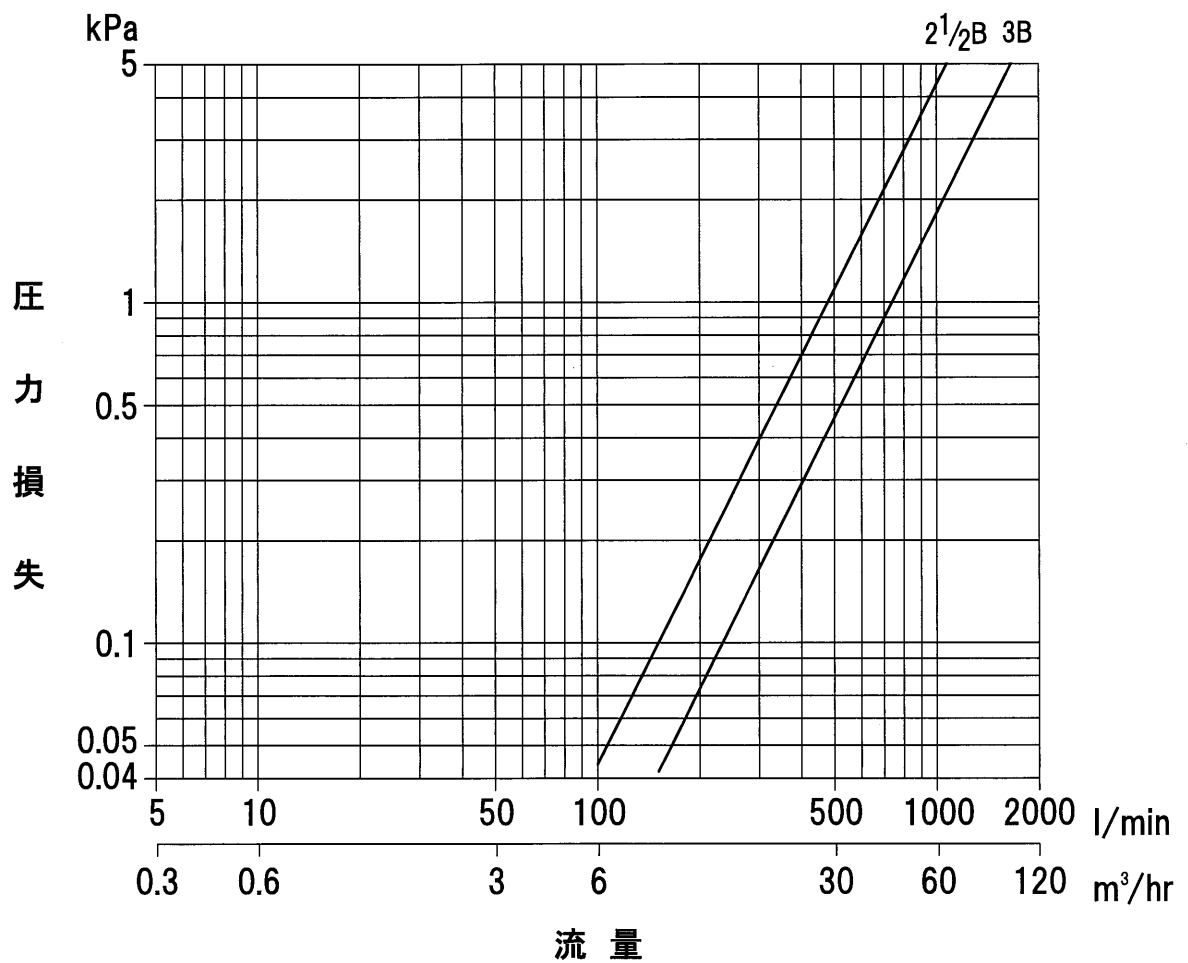
圧力損失—流量線図
