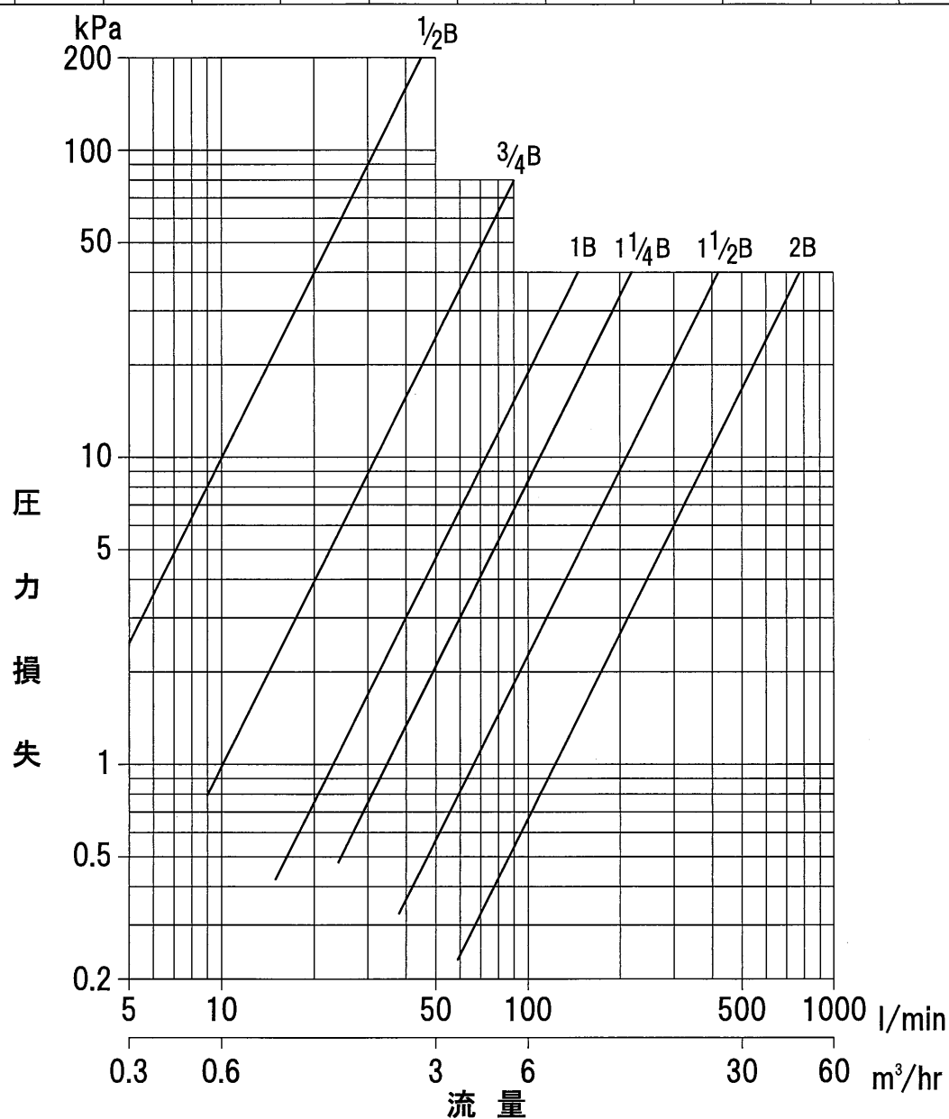
圧力損失—流量線図
